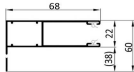
Führungsschiene A 14
