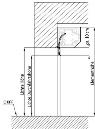
Linksroller Montage vor der Laibung
