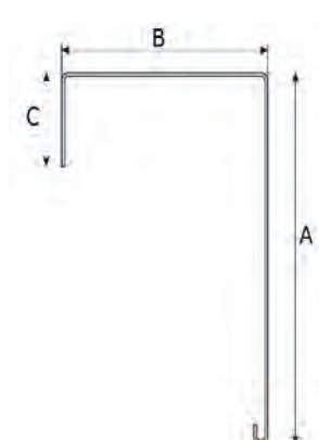
Blende F21
