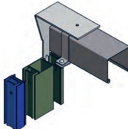
System ohne Blende STF 2
