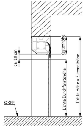
Linksroller Montage in der Laibung
