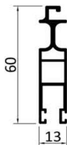
Flügelprofil ST
