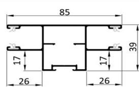
Doppelführungsschiene DF A 15-CR
