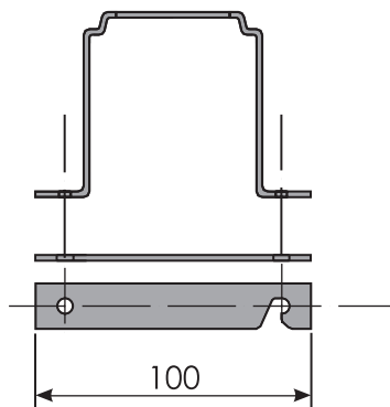
Halter Nr. 3 (K / M / L)
