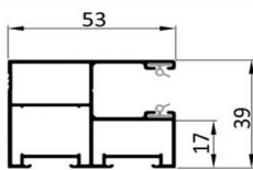
Abstandsführungsschiene A 16-CR nur bei Kastengröße 138 - 180 verwendbar clipsbar und schlagregensicher
