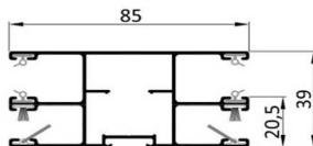
Doppelführungsschiene für Insektenschutz DF A 20-CR
