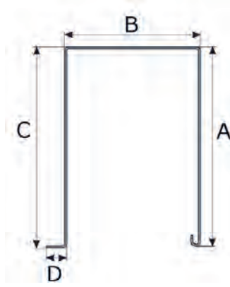
Blende F32
