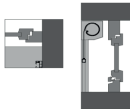
Rechtsroller
