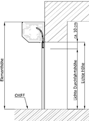
Linksroller Montage vor der Laibung
