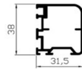
Rahmenprofil RT-50
