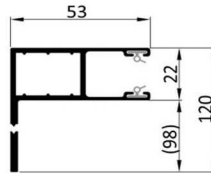
Führungsschiene A 12
