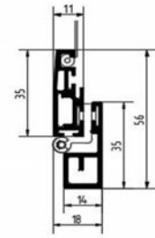
DR-B
