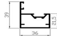
Rahmenprofil RT-50
