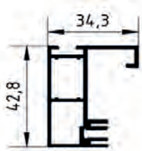
A31-G
