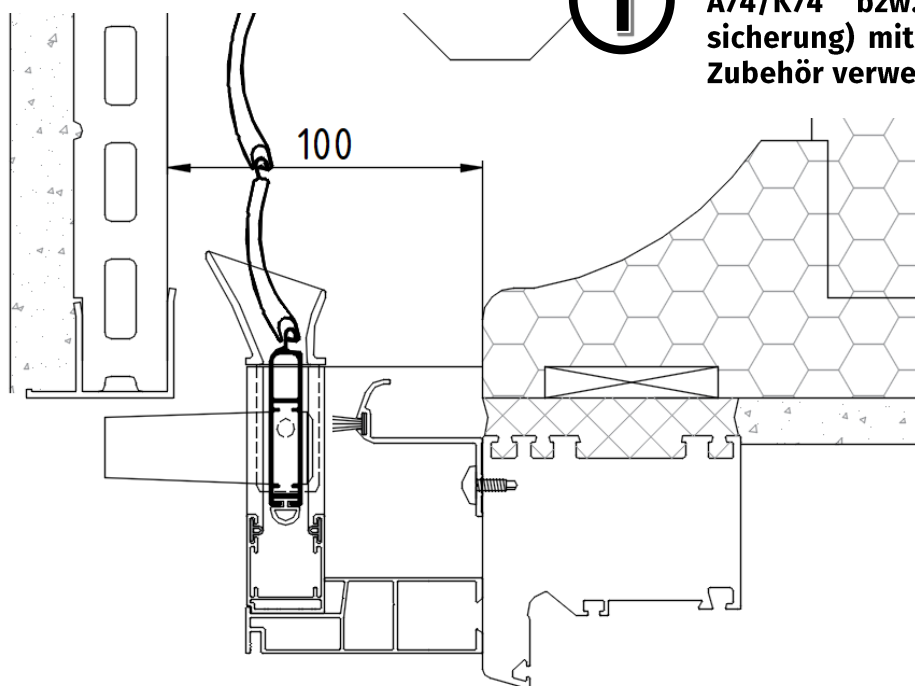
V2: Schachttiefen ab 95 mm (negativer Einlauf)
