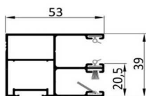
Insektenschutzführungsschiene A 20-CR (ohne Aufpreis)
