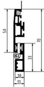
RT-V
