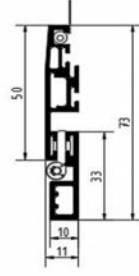
DR-V
