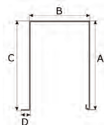
Blende F32
