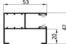
Abstandsführungsschiene A 8-20 20 mm Abstand
