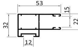
Führungsschiene A 3-10-CR clipsbar und schlagregensicher 10 mm Abstand
