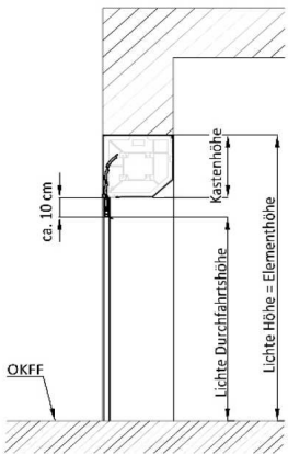
Linksroller Montage in der Laibung
