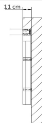
Wandbefestigung wenn < 13,5 cm
