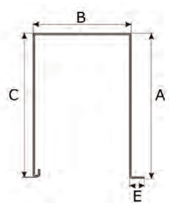
Blende F33
