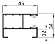
Abstandsführungsschiene A 5-12 12 mm Abstand
