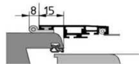
RT-V ohne Rahmen Flügelprofil unten (siehe Kap. 8 Aufmaß- und Bestellhilfe)
