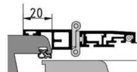
Pendeltür mit Rahmen
