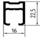
Z-Profil
