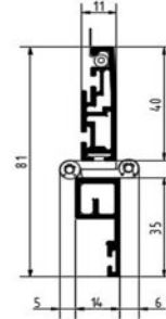
Pendeltür
