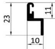
Z-Profil
