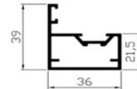
Rahmenprofil RT-50
