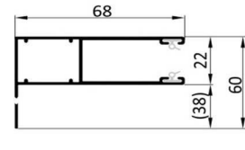
Führungsschiene A 14
