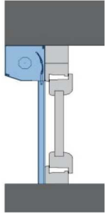
Standardführungsschiene A 3
