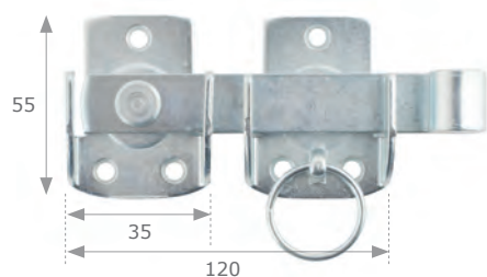
Klappladenverschluss mit 4 Nasen + Zugring
